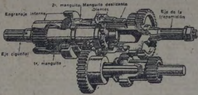
Fig. 2a. — Ejes y engranajes del nuevo tipo de caja de cuatro velocidades adelante, la cual está siendo ensayada en América. La máxima velocidad se obtiene directamente y la "tercera" se obtiene por engranajes internos silenciosos.
