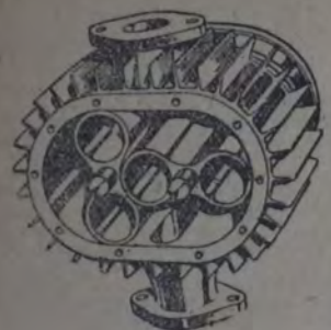
Fig. 2b. — Vista especial del compresor Plesco, el cual es uno de los más empleados para los propósitos de la sobrealimentación en los modernos motores
