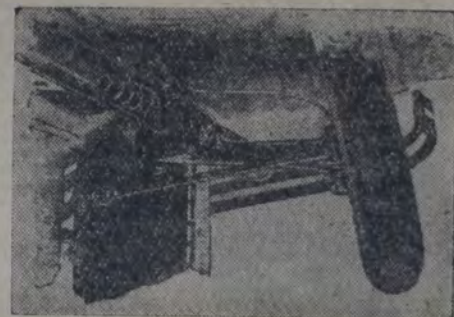
Fig. 5a. — Suspensión y muellejo independiente de las ruedas: El sistema H. L. L. representado en la fig. 5, el cual acaba de sufrir una serie de pruebas en Francia, con todo éxito: cada rueda va suspendida por un brazo oscilante trabajando contra un fuerte resorte en espiral colocado en el interior del extremo del chasis tubular.
