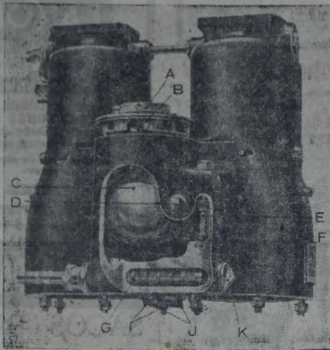
A. Tornillo de mano de sujeción de la tapadera. — B. Mango para apretar la tapadera. — C. Flotador. — D. Eje del flotador. — E. Aguja de la válvula. — F. Cámara de la aguja. — G. Filtro de entrada de la gasolina. — H. Tapones de los compensadores. — I. Tapones de los surtidores o inyectoras. — J. Tapón del pozo del filtro. — K. La entrada de la gasolina puede hacerse, indistintamente, por uno y otro lado de este pozo
