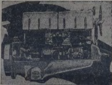
Fig. 4a. — Motor Diesel, en el cual sólo el aire se comprime, el combustible pesado se inyecta por medio de bombas al centro de la cámara de combustión, donde se inflama por el calor del aire comprimido, sin necesidad de aparatos provocadores de la ignición.
